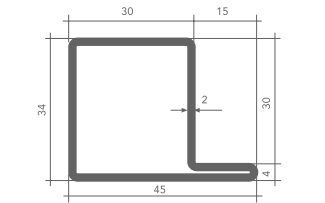
L30-34x15x2 • 55%
