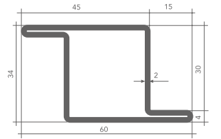
Z30-34x15x2 • 55%
