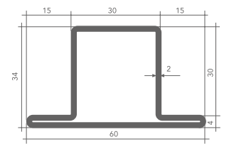
T30-34x15x2 • 55%
