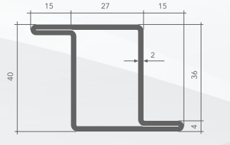
Z27-40x15x2 • 50%
