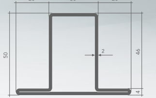
T30-50x20x2 • 45%
