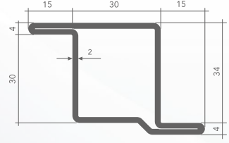
ZD28-34x15x2 • 55%
