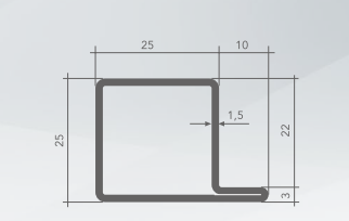
L25x25x10x1,5 • 60%
