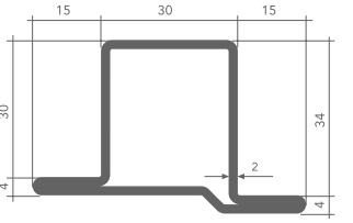
TD28-34x15x2 • 55%
