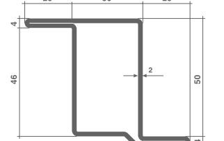
ZD30-50x20x2 • 45%
