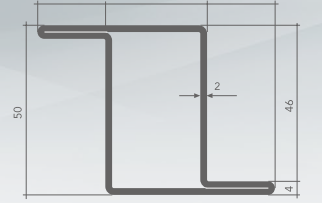
Z30-50x20x2 • 45%
