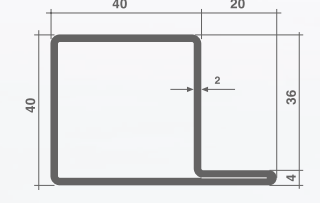
L40x40x20x2 • 50%
