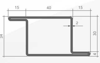
Z40x34x15x2 • 50%
