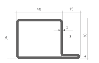
L40-34x15x2 • 50%
