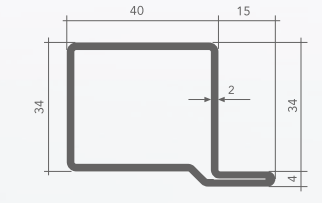
LD40x34x15x2 • 50%
