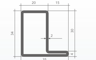
L20-34x15x2 • 60%
